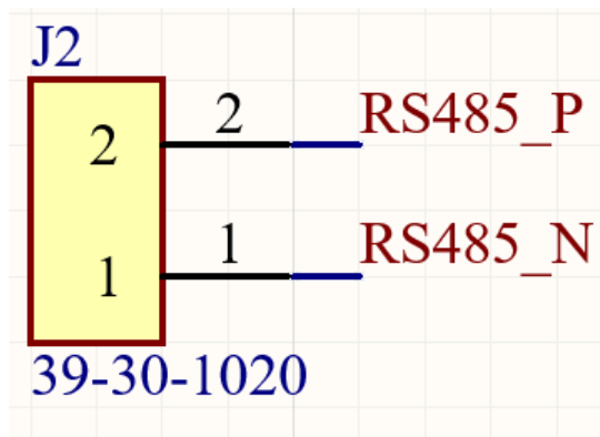
Schemat i fizyczny wygląd złącza J2.
