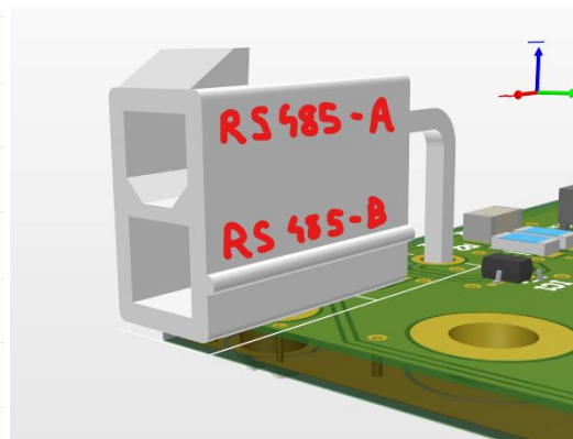
Schemat i fizyczny wygląd złącza J2.
