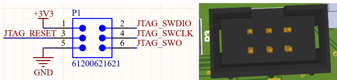
Schemat i fizyczny wygląd złącza P1 (podpisane piny od spodu płytki)
