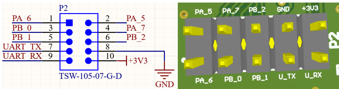
Schemat i fizyczny wygląd złącza P2
